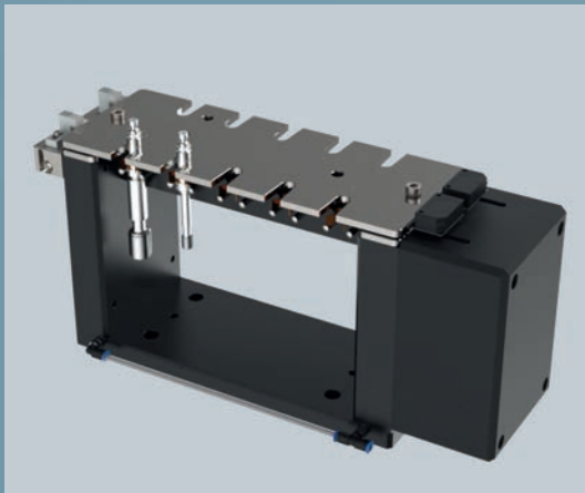
Automatisiertes Lehrenmagazin für bis zu 10 Lehreneinsätze
